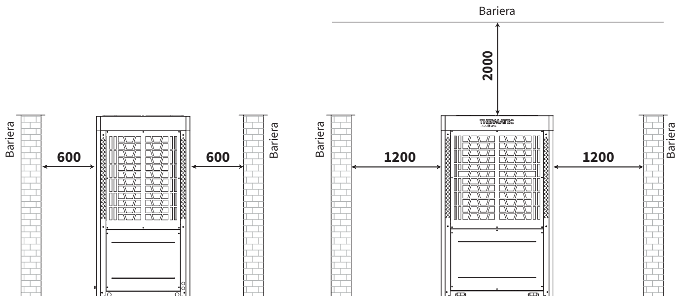
Rysunek 3. Odległość przeszkody w kierunku poziomym i pionowym (mm)
